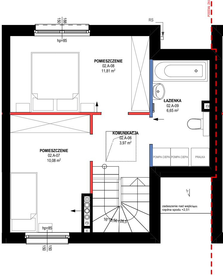
RZUT 1 PIĘTRA
